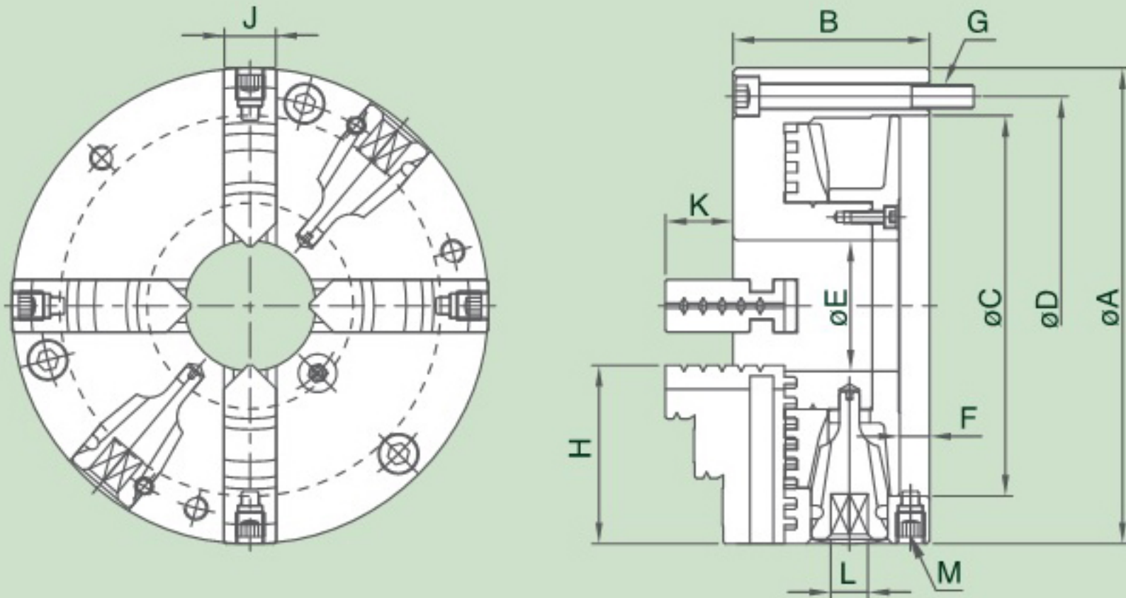
尺寸圖 » Dimensions
